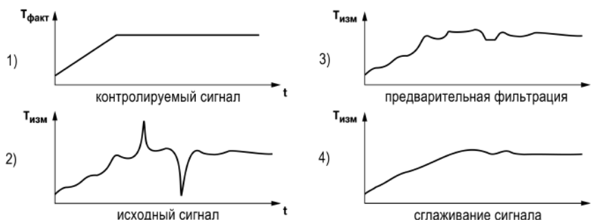
Рисунок 7.7 – Работа фильтров
